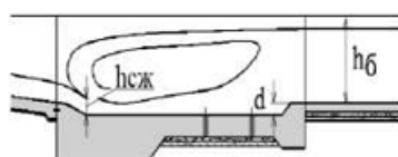
Водобойный колодец
