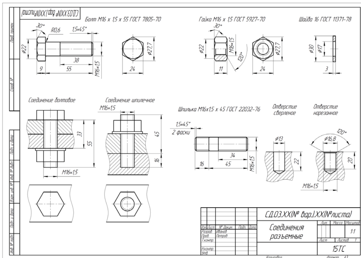
Рис. 6. Соединения разъемные резьбовые.
