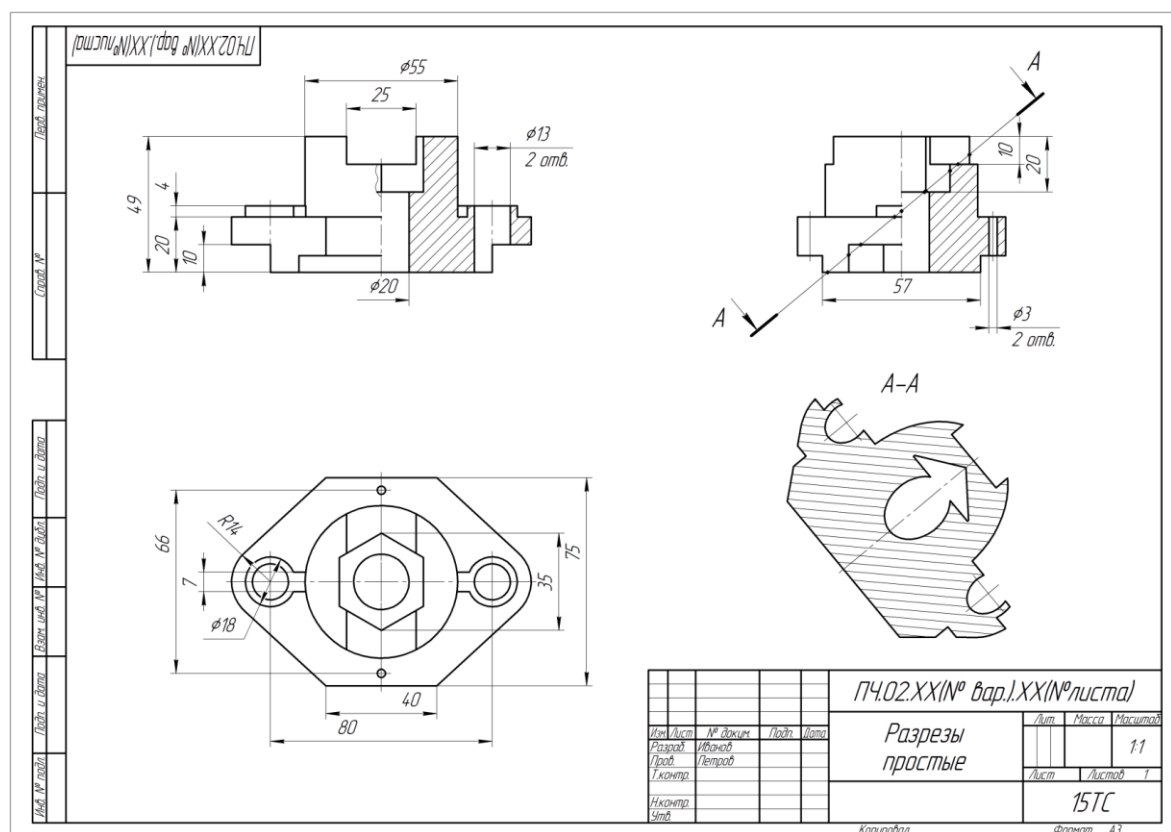
Рис. 4. Простые разрезы.
