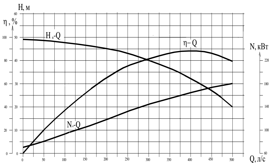
Характеристика насоса Д-1000 - 40 (14НДс), n = 980 об/мин
