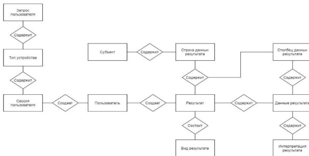
Рисунок 4 – Концептуальная модель базы данных
