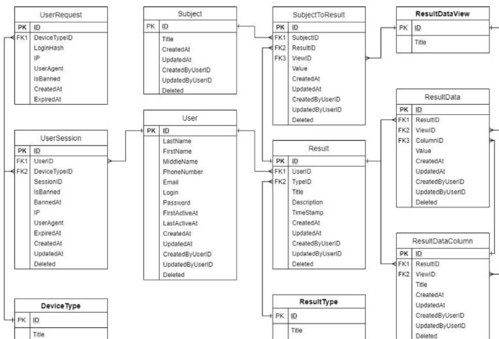
Рисунок 4 – Концептуальная модель базы данных
