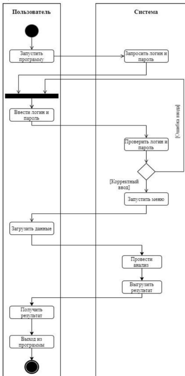
Рисунок 2 – Диаграмма деятельности пользователя в системе
