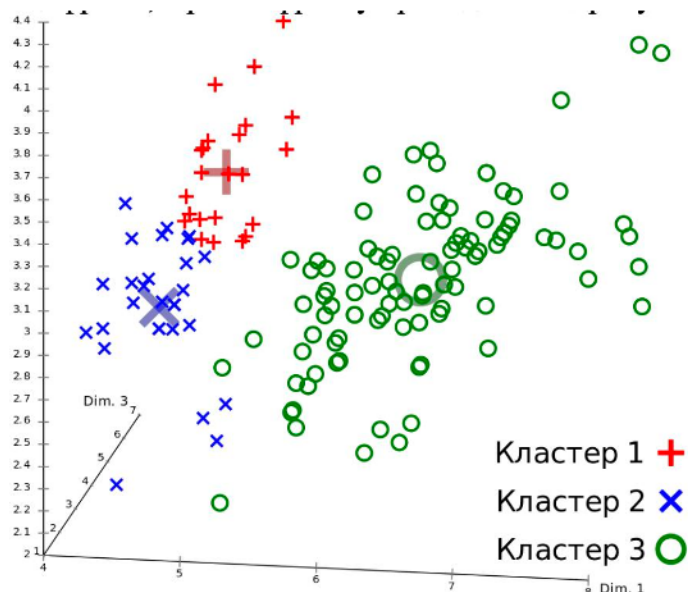
Рис. 3.1 – Метод k-средних
