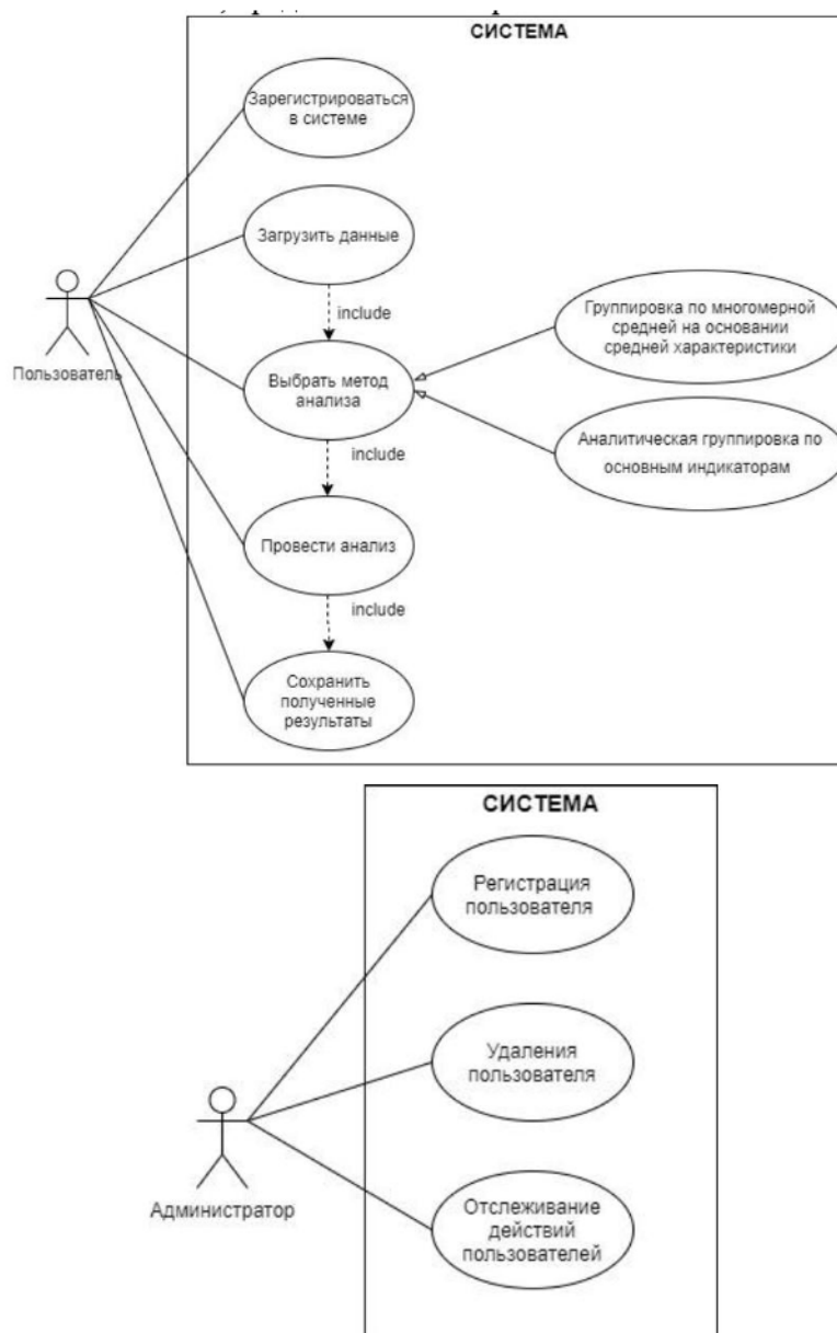
Рисунок 1 – Варианты использования системы
