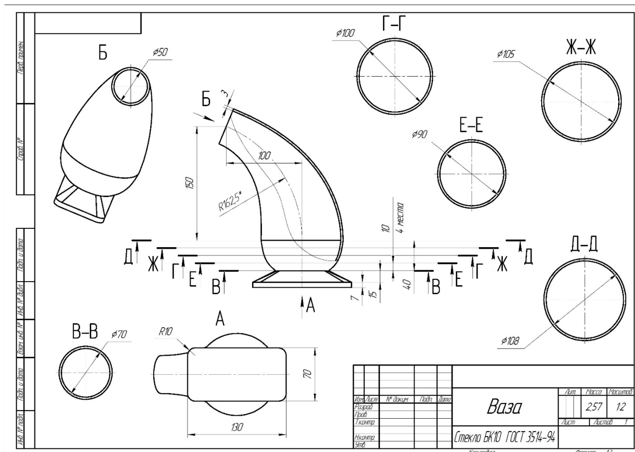
Рис. 4. Моделирование деталей по сечениям
