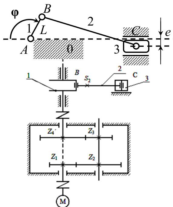
Структурные схемы привода и дополнительного механизма
