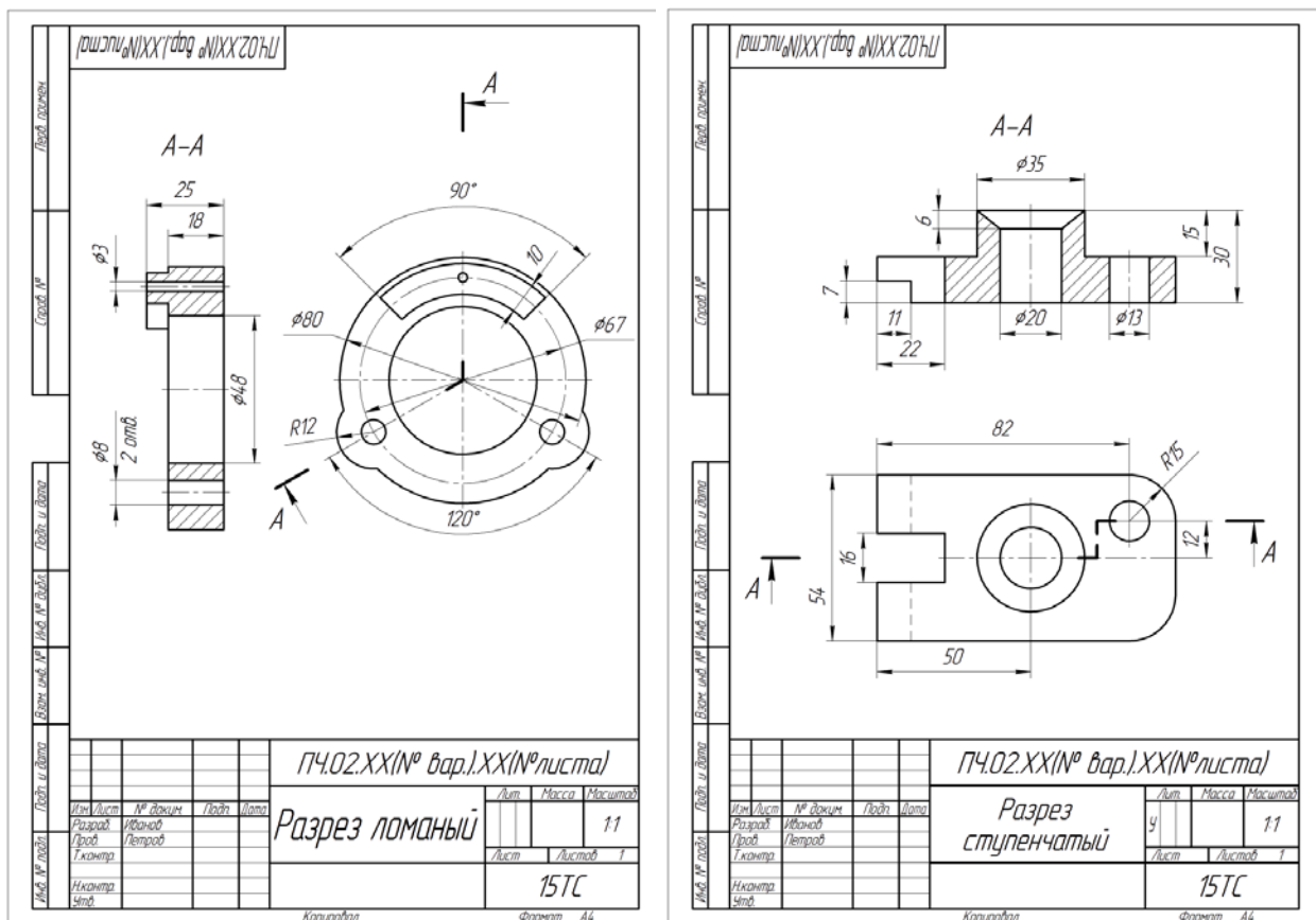
Рис. 5. Сложные разрезы.
