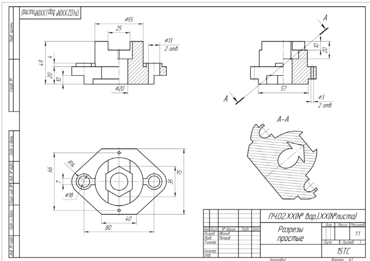
Рис. 4. Простые разрезы.
