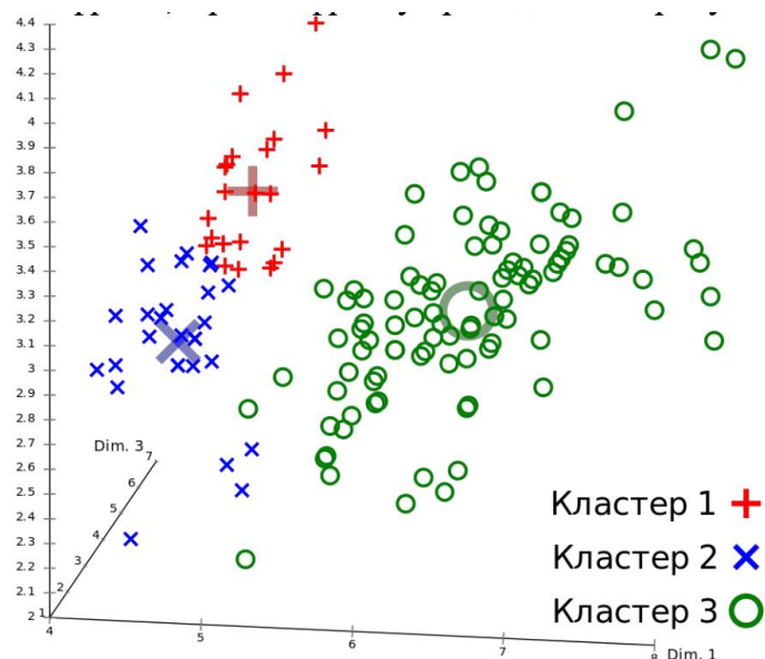
Рис. 3.1 – Метод k-средних
