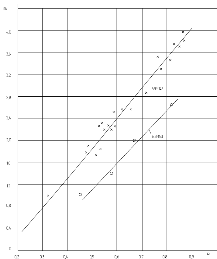
Рисунок 2.2 – Зависимость параметров от номинальной степени заряженности аккумуляторных батарей 6ЭМ145 и 6ЭМ60
