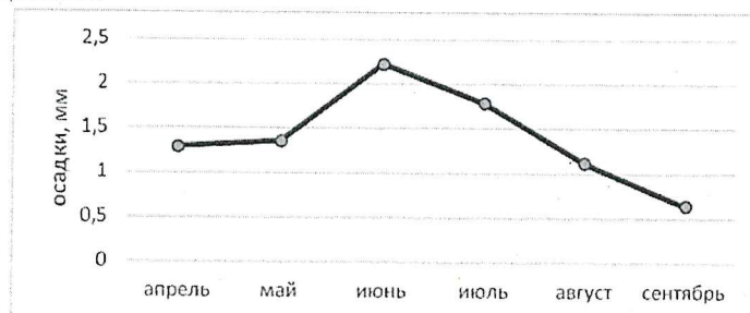
Рис. 3.1 Среднее количество выпавших осадков
