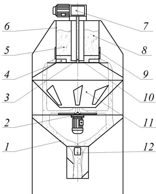
Рисунок 1 - Схема дозатора-смесителя сыпучих кормов:
